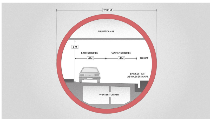
Normalprofil 2. Röhre Gotthard-Strassentunnel gemäss Detailprojekt
