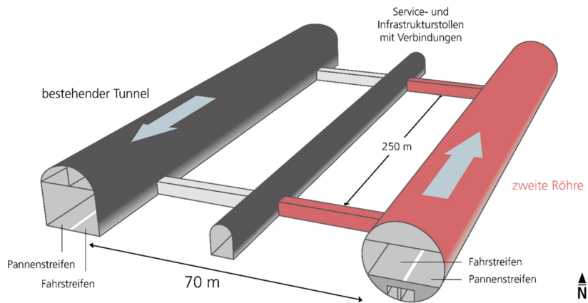
Konzept Gotthard-Strassentunnel mit 2. Röhre (Neubauteil in Rot)
