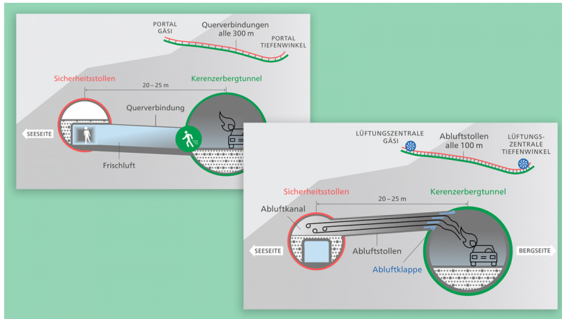
Infografiken zu den Massnahmen im Sicherheitsstollen
