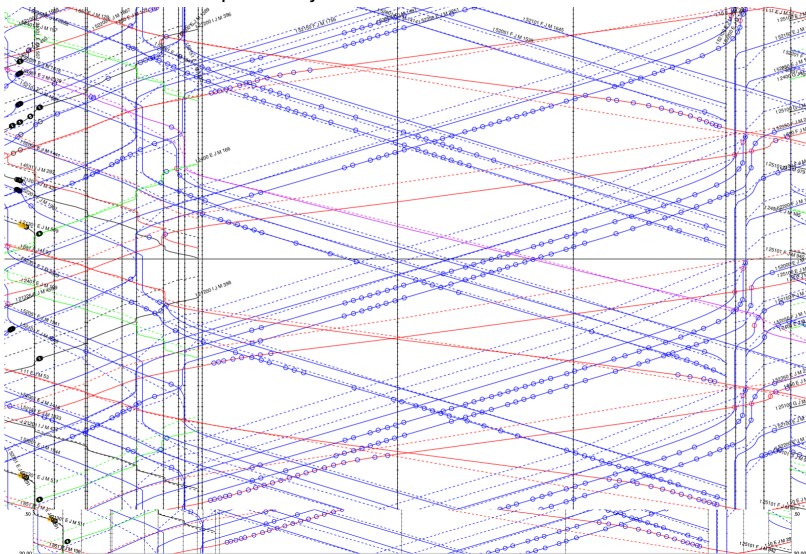
Bildfahrplan für den Streckenbereich des Gotthard-Basistunnels in einer Simulation. (Für vergrösserte Ansicht, Bild anklicken.)
