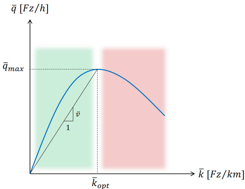
Theoretische Form des MFD: Abhängigkeiten von mittlerer Fahrzeugdichte k (x-Achse) und mittlerem Verkehrsfluss q (y-Achse).
