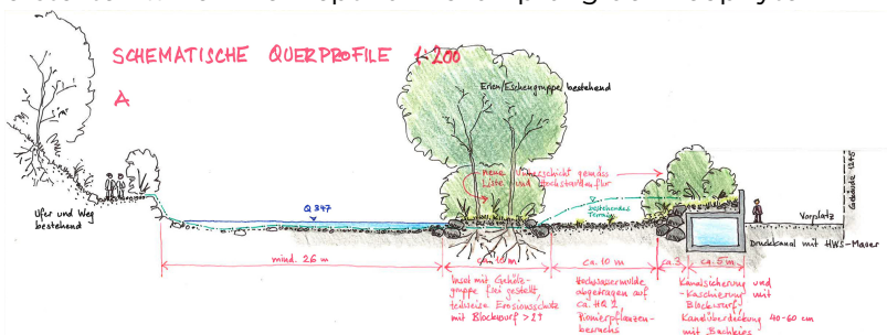
Schematisches Querprofil zum ökologischen Ausgleich und Ersatz im Bereich der Hochwasserinsel.
