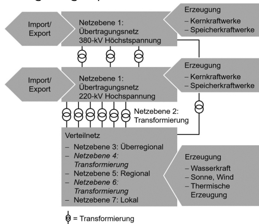
Übersicht der Schweizer Stromversorgung
