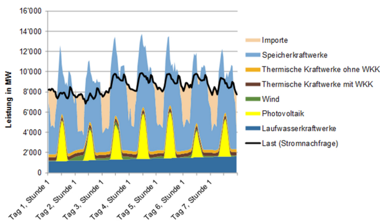
Referenz: stundengenaue Modellierung einer Woche in der zweiten Hälfte des Februars 2011/12
